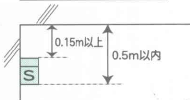
壁に設置する場合
