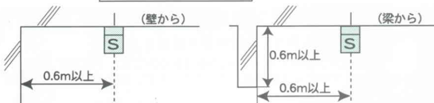
天井に設置する場合
